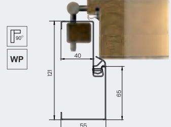
aluminiowy ALU S15/75 3P
