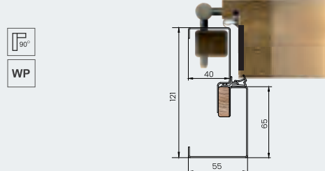
aluminiowy ALU NT/75 3P
