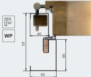
aluminiowy ALU NT/75 3P
